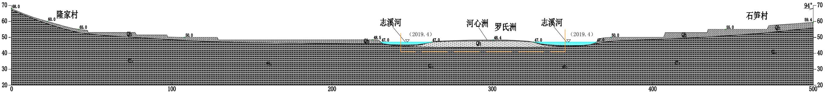
益阳市赫山区志溪河禁采区1河段C线地质剖面图
