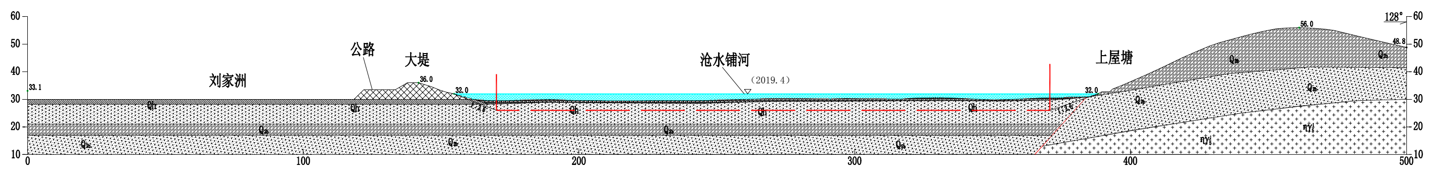
益阳市赫山区侍郎河哑河采区（2可采段）E线地质剖面图
