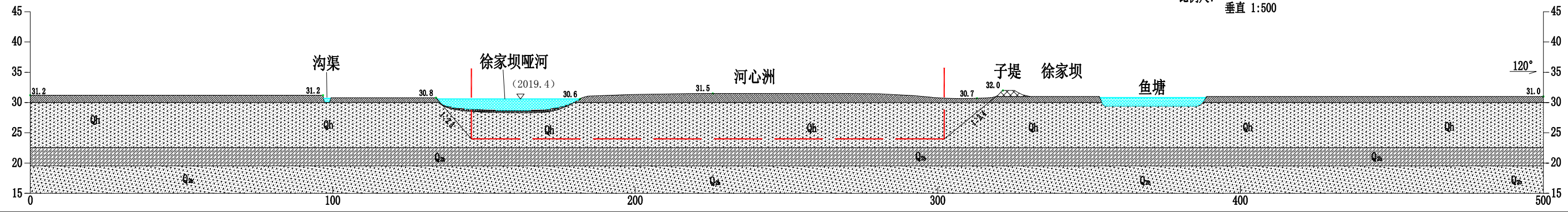
益阳市赫山区徐家坝哑河采区1（可采段）F线地质剖面图
