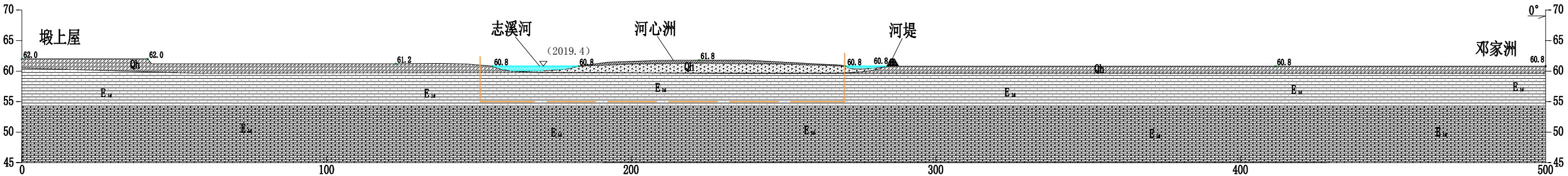
益阳市赫山区志溪河保留区1河段B线地质剖面图
