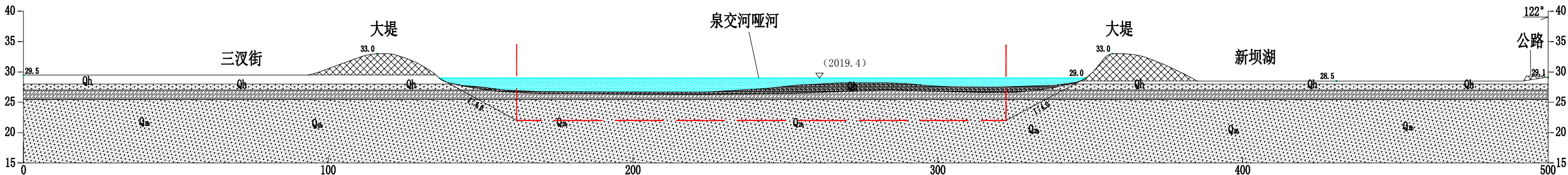
益阳市赫山区张芦渠采区（3可采段）I线地质剖面图
