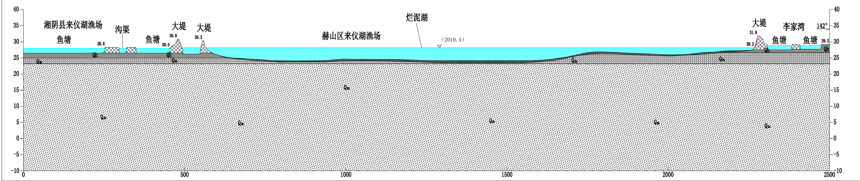
益阳市赫山区鹿角湖禁采区K线地质剖面图
