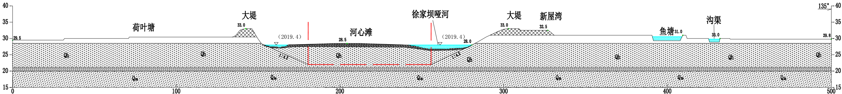
益阳市赫山区泉交河哑河采区2（可采段）H线地质剖面图
