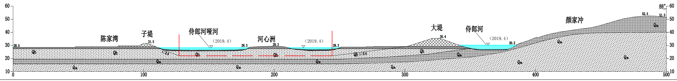
益阳市赫山区徐家坝哑河采区1（可采段）F线地质剖面图
