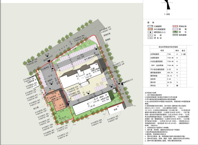
益阳市公安局八字哨派出所业务用房建设项目-总平面图 1:500
