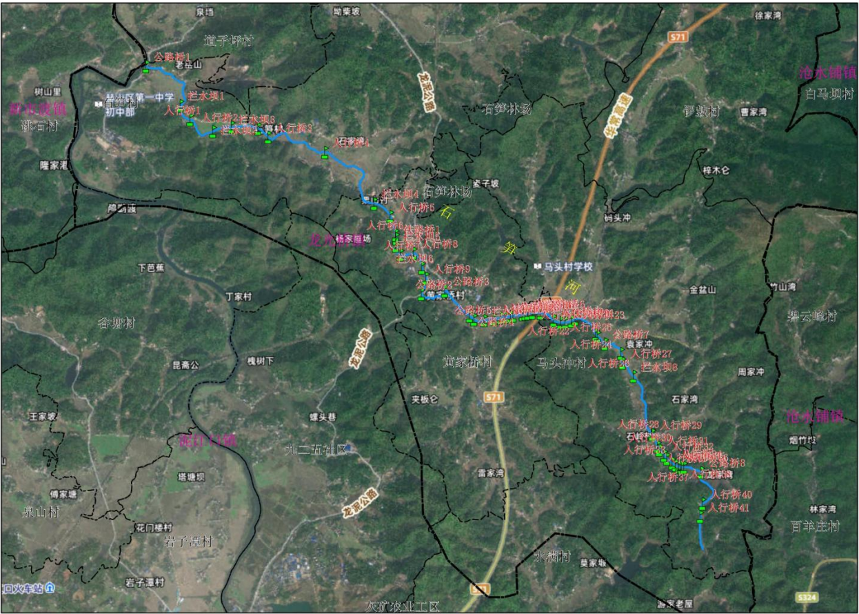
图 2.3-1 石笋河涉河建筑物分布示意图
