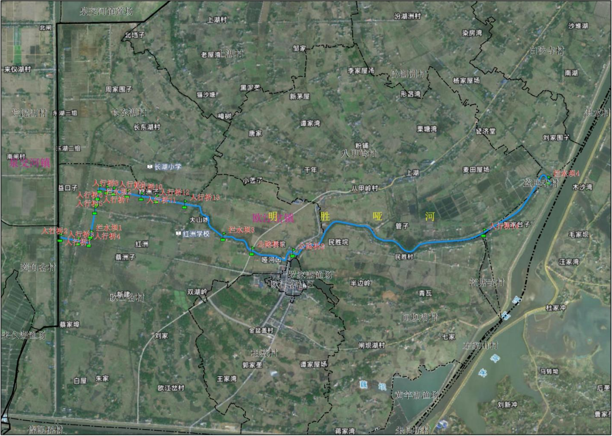
图 2.3-1 明胜哑河涉河建筑物分布示意图
