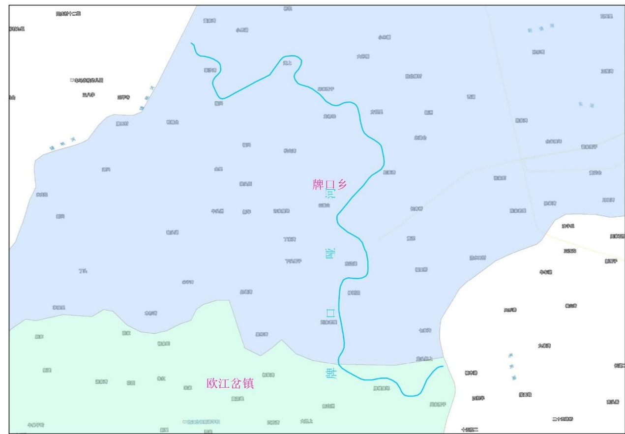
图 2.1-1 牌口哑河地理位置图
