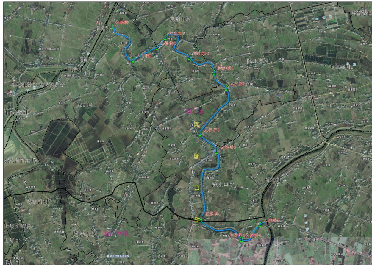
图 2.3-1 牌口哑河涉河建筑物分布示意图
